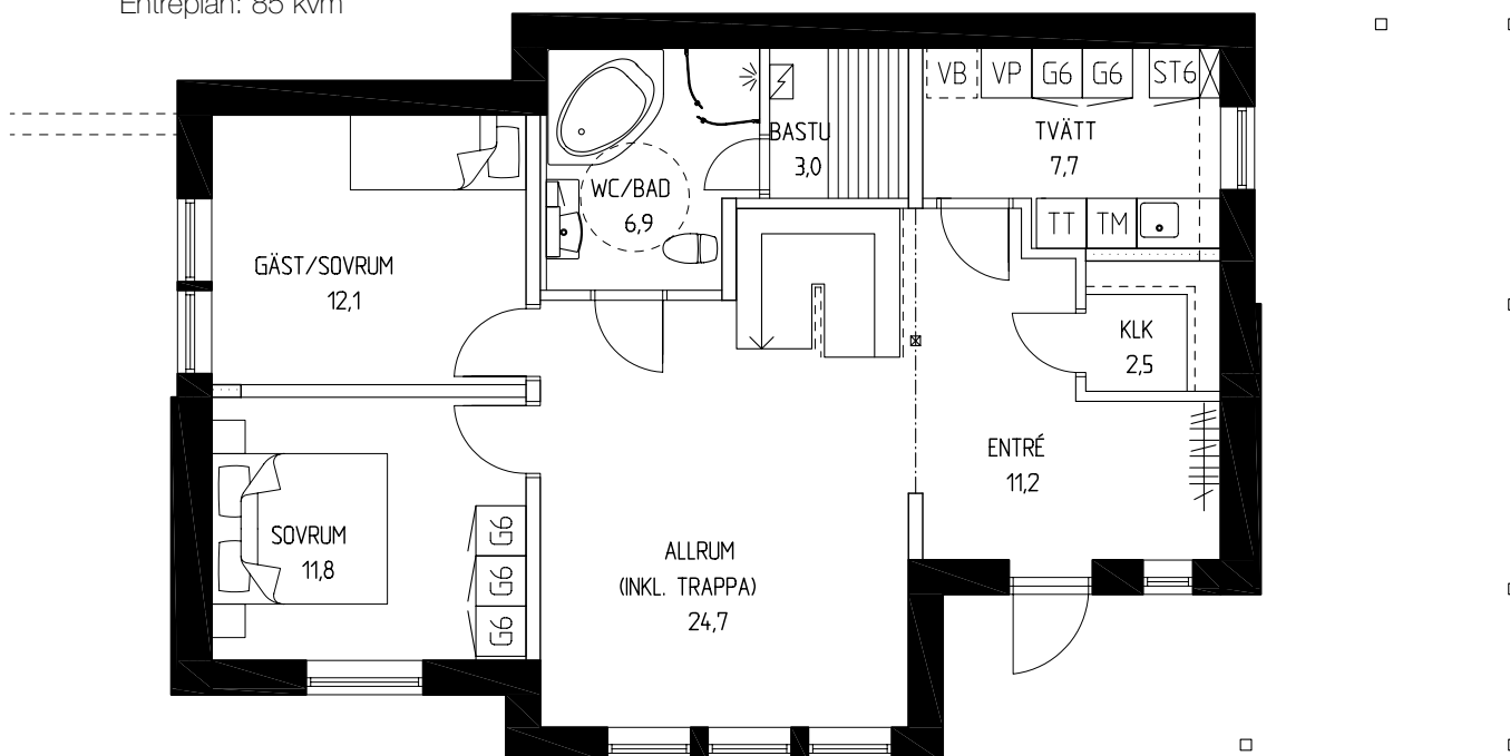
Entréplan: 85 kvm
